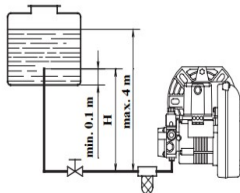
Εικόνα 13.2 Μονοσωλήνια τροφοδοσία
