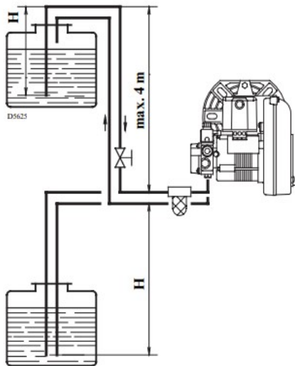
Εικόνα 13.1 Δισωλήνια τροφοδοσία
